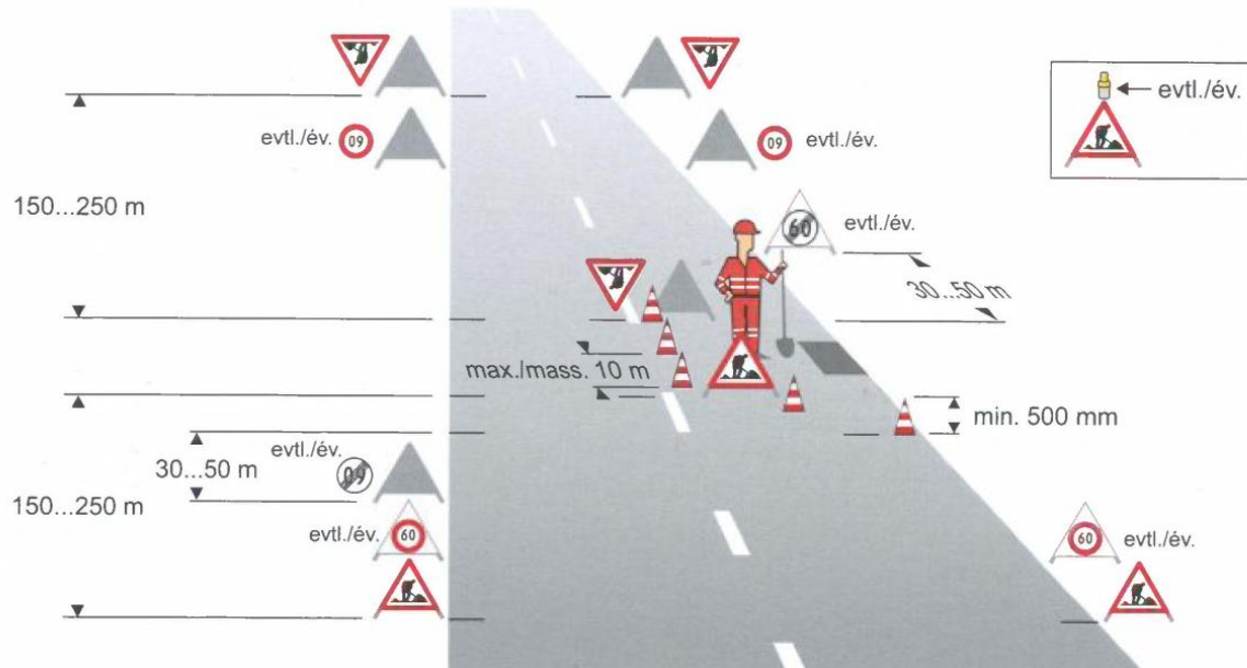
Abbildung 2 Kurzbaustelle, Hindernis auf der Fahrbahn ausserorts, Bild VSS 40 886 (2019)
